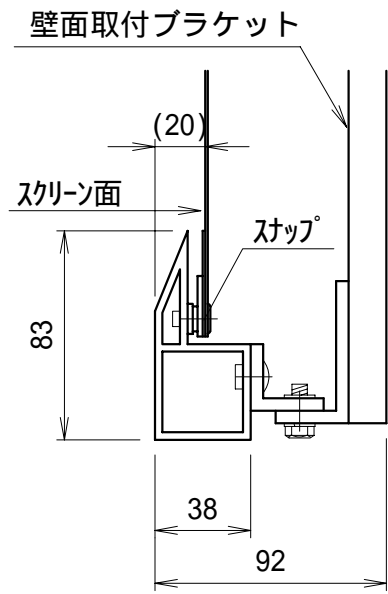
① 断面図 S=1/3
